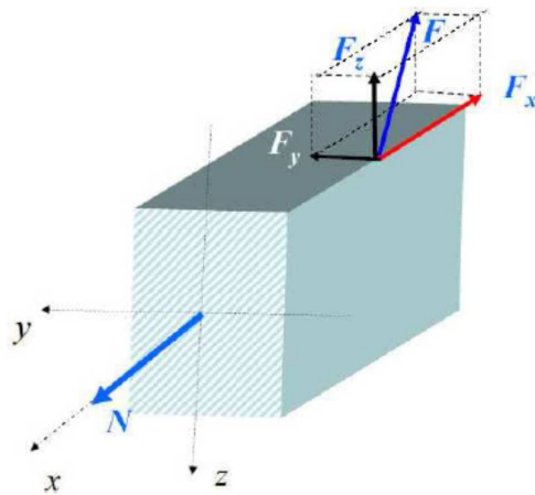
Joonis 2.2: Pikijõud
