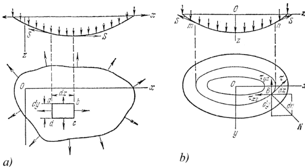
Joonis 8.5: Põikkoormusega koormatud ühtlaselt tõmmatud membraan — a); deformeerunud membraani samaläbipainde jooned — b). NB! \tau_{yz} = \tau_{zy}
